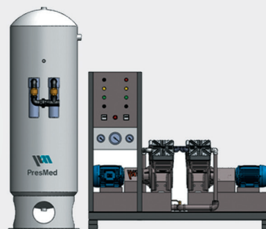
Central Geradora de Vácuo Clínico Duplex
